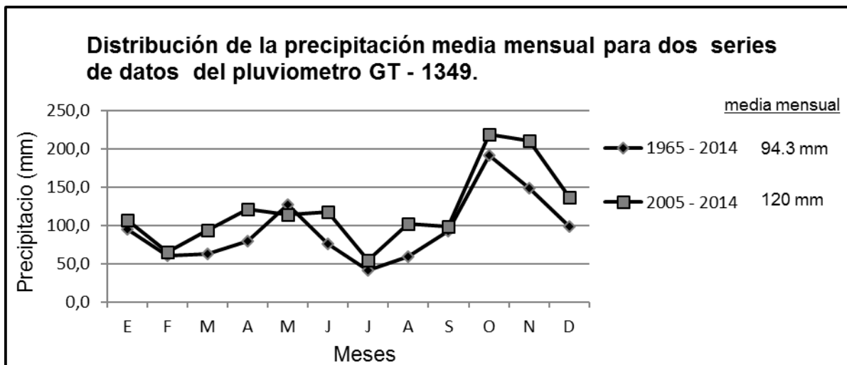
Figura 2: Distribución de la media mensual de los acumulados de precipitaciones para las series de datos de los periodos años 1965 – 2014 y años 2005 - 2015 del pluviómetro GT- 1349 de Lindero en Maisí.
