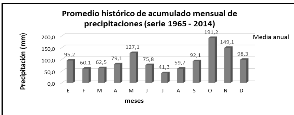
Figura 1: Distribución de la media mensual de los acumulados de precipitaciones para la serie histórica 1965 – 2014 del pluviómetro GT- 1349 de Lindero en Maisí.
