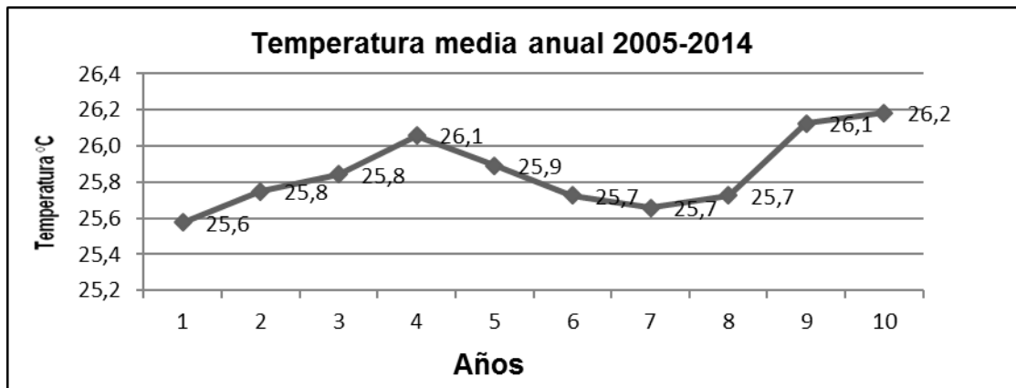
Figura 3: Distribución de la temperatura media anual durante el periodo 2005 – 2014.
