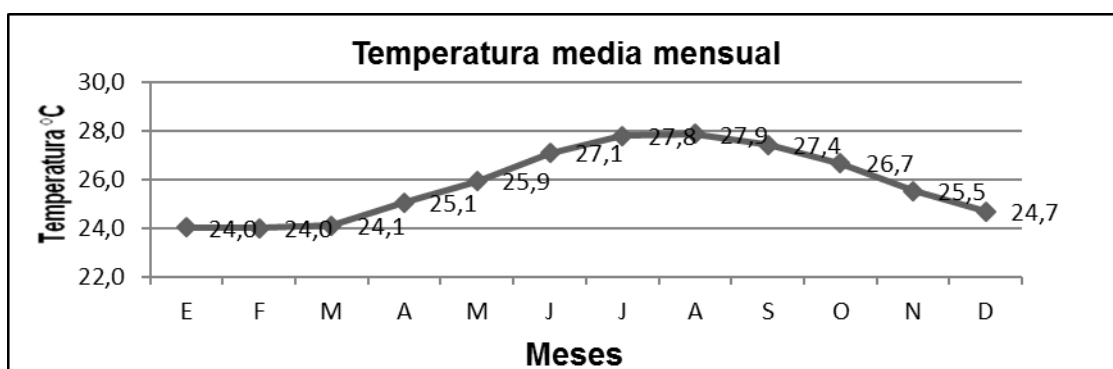
Figura 4: Distribución de la temperatura media mensual durante el periodo 2005 – 2014.
